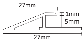
RV5 27-A alumínio versão com adesivo
