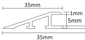
RV5 35-F alumínio versão furada
