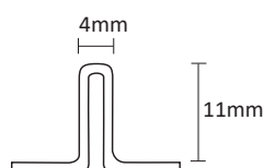
DS4 Alumínio
