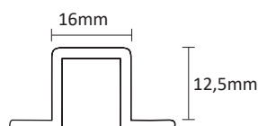
DS16 Alumínio
